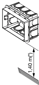
Scatola 503 Boîtier 503
