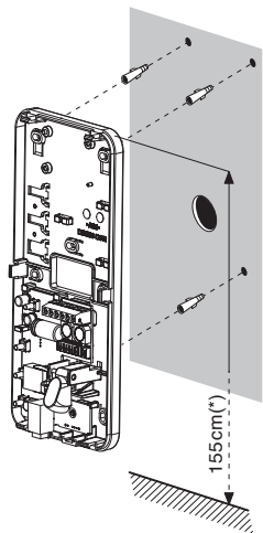
Scatola 503 Boîtier 503
