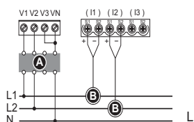
1PH3W L-L-N
