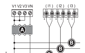
1PH4W multi L-N 3LVCS
