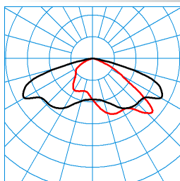
Jovie 70-AB7L-ML-LR/165-240-730 24G1 ET (CLO end value) TX271491 ■ C0 - C180 ■ C90 - C270 DIN 5040: A30 UTE: 1,00 G CEN Flux Code: 35 73 97 100 100
