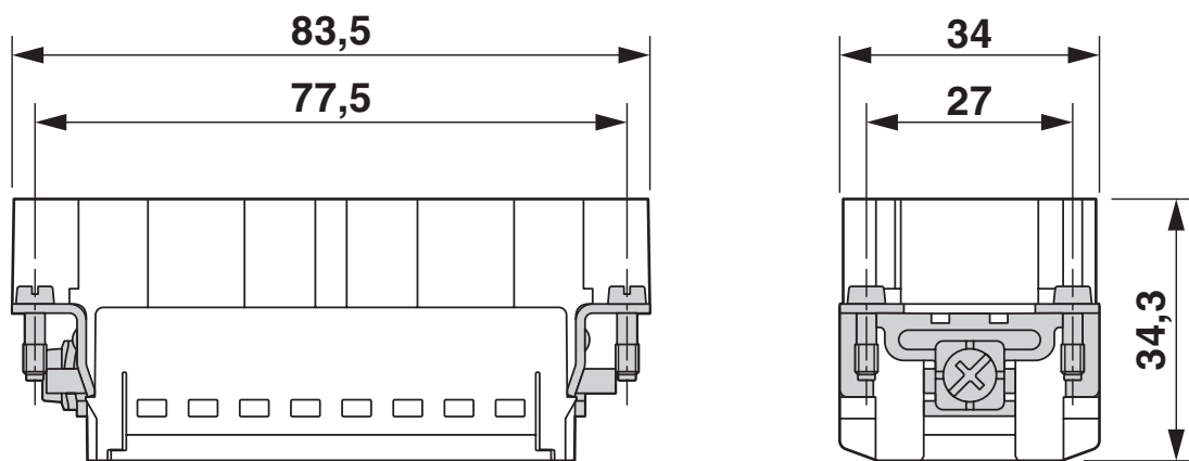
Dessin coté
