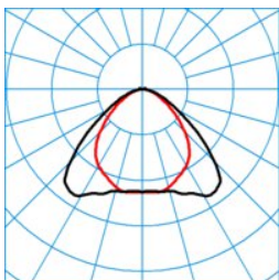
ELINE LVW55-140 ML 840 L225 0 50 ■ C0 - C180
