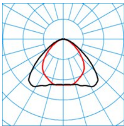
ELINE LVW55-140 ML 840 L225 2 50 ■ C0 - C180
