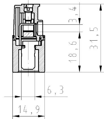
Schnitt A-A section A-A
