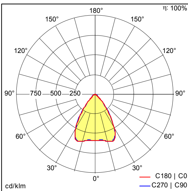
D46452_CR2_M17k-840_PC_WB_LDO.Idt
