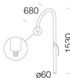
1473 Bras courbé
