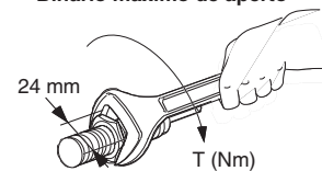
XU-N18 : T = 15 Nm XU-P18 : T = 5 Nm
