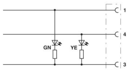
Schaltplan
