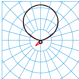
LuceoS S-T PAW-IL 300-830 03(LEO2) TX373163 ■ C0 - C180 ■ C90 - C270 DIN 5040: E03 UTE: 0,08 D + 0,91 T CEN Flux Code: 53 86 96 8 100 49 82 98 92
