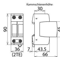
Dimensions DG M TT 2P 275 NL
