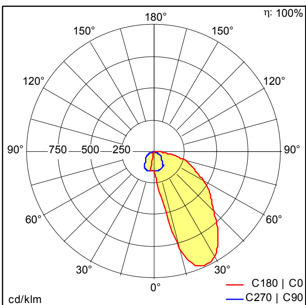
D34983AA_TECTON_C_LED3700-865_L1000_WW_EVG_WH.Idt
