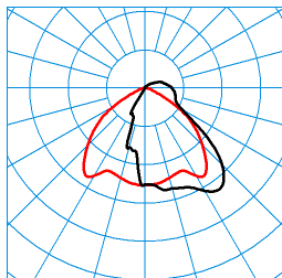
TX044704 DIN 5040: A40 UTE: 0,92 D + 0,08 T ■ C0 - C180 ■ C90 - C270
