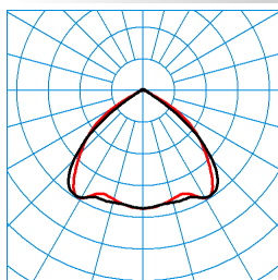
TX040451 UGR I = 21.9 UGR q = 20.9 DIN 5040: A40 UTE: 0,98 C + 0,02 T ■ C0 - C180 ■ C90 - C270
