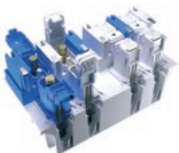
Détail connectique
