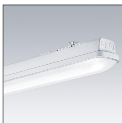
Luminaire étanche LED AQFPRO L LED4300-840 PC WB HF 96630756
