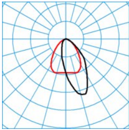
ELINE LAN40-110 ML 830 L150 4 20 ■ C0 - C180
