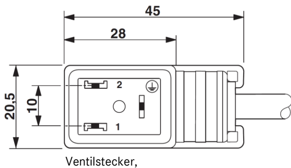
Maßzeichnung
