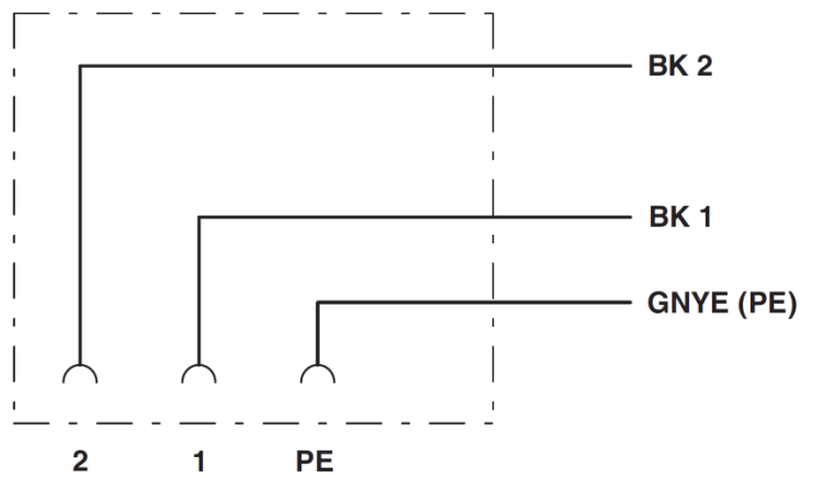
Schaltplan
