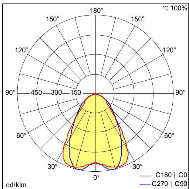
D46285AA_TRINOS_5000-840_L1000_WB_LDE_WH.Idt
