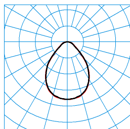
ArmoFit M48 PW19 53-840 ET TWW + ArmoFit Sky M48-TS ZER TX426325
