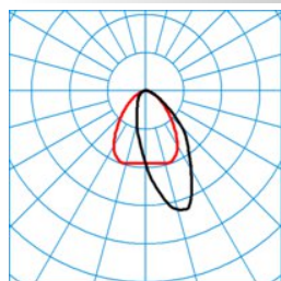
7850 LAN60 840 L225 1 50
