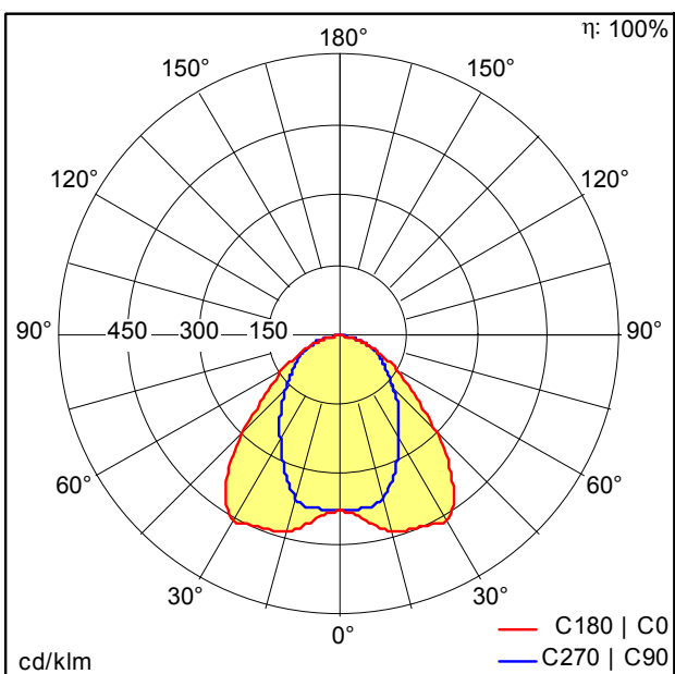
D41246AA_TECTON_C_LED5200-840_L1000_VWB_LDE_BK.lgt
