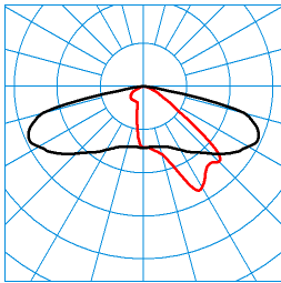
Jovie 50-AB2L-LRA/1000-740 2G1 ET (CLO end value) TX300501 ■ C0 - C180 ■ C90 - C270 DIN 5040: A30 UTE: 0,98 l CEN Flux Code: 34 70 96 100 98
