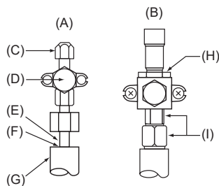
(A) Válvula <Lado de líquido> (B) Válvula <Lado de gas> (C) Puerto de servicio (D) Sección Abierto/Cerrado (E) Tubo local (F) Sellado, igual para lado de gas (G) Cubierta del tubo (H) No utilice una llave aquí. Podría producirse una pérdida de refrigerante. (I) Utilice dos llaves aquí.
