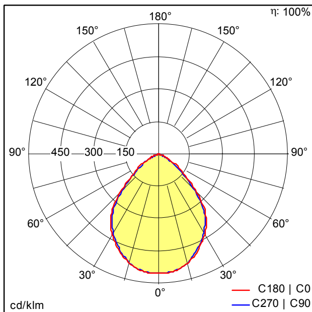
D43600AA_CLEVO_MSC_6800-840_L3080_LDO_WH_WHM.Idt
