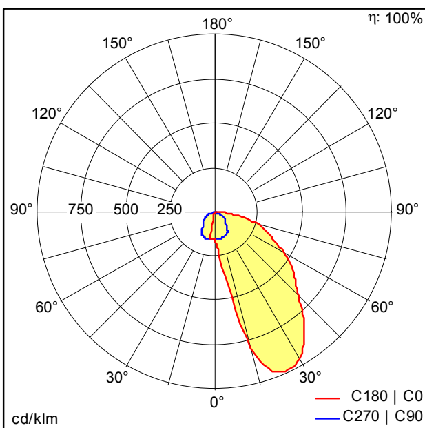
D34983AA_TECTON_C_LED8000-830_L1500_WW_LDE_SR.Idt
