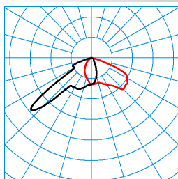
LIQ 50N-FL1L/5600-740 6G1 ET (CLO end value) TX278272 ■ C0 - C180 ■ C90 - C270 DIN 5040: A40 UTE: 1,00 F CEN Flux Code: 43 84 100 100 100
