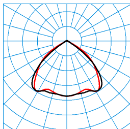
TX053214 UGR I = 20.7 UGR q = 19.5 DIN 5040: A40 UTE: 0,98 C + 0,02 T ■ C0 - C180 ■ C90 - C270
