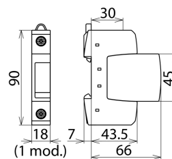
Dimensions DK 25
