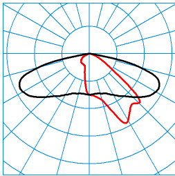
Jovie 50-AB2L-LRA/4200-740 4G1 ET (CLO end value) TX300743 ■ C0 - C180 ■ C90 - C270 DIN 5040: A30 UTE: 1,00 G CEN Flux Code: 34 71 96 100 100
