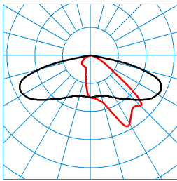
Jovie 50-AB2L-LRA/4200-740 4G1 ET TX068567 ■ C0 - C180 ■ C90 - C270 DIN 5040: A30 UTE: 1,00 G CEN Flux Code: 34 71 96 100 100
