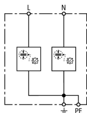
Schéma de principe du circuit DSH TN 255
