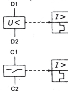
LA1-LC07●● (TRIP. Déclenché)
