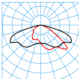
Jovie 70-AB7L-ML/165-240-740 24G1 ETDD (CLO end value) TX271528 ■ C0 - C180 ■ C90 - C270 DIN 5040: A30 UTE: 1,00 G CEN Flux Code: 35 73 97 100 100
