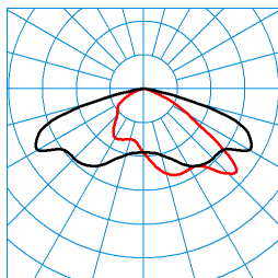
Jovie 70-AB7L-ML/165-240-740 24G1 ETDD (24000 lm) TX068716 ■ C0 - C180 ■ C90 - C270 DIN 5040: A30 UTE: 1,00 G CEN Flux Code: 35 73 97 100 100
