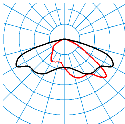
Jovie 70-AB7L-ML/165-240-740 24G1 ETDD (20000 lm) TX068715 ■ C0 - C180 ■ C90 - C270 DIN 5040: A30 UTE: 1,00 G CEN Flux Code: 35 73 97 100 100
