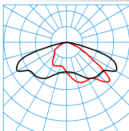
Jovie 70-AB7L-ML/165-240-740 24G1 ETDD (16500 lm) TX068714 ■ C0 - C180 ■ C90 - C270 DIN 5040: A30 UTE: 1,00 G CEN Flux Code: 35 73 97 100 100
