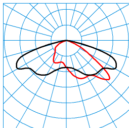
Jovie 70-AB7L-ML/5600-6800-740 8G1 ETDD (6200 lm) TX068721 ■ C0 - C180 ■ C90 - C270 DIN 5040: A30 UTE: 1,00 G CEN Flux Code: 34 71 96 100 100
