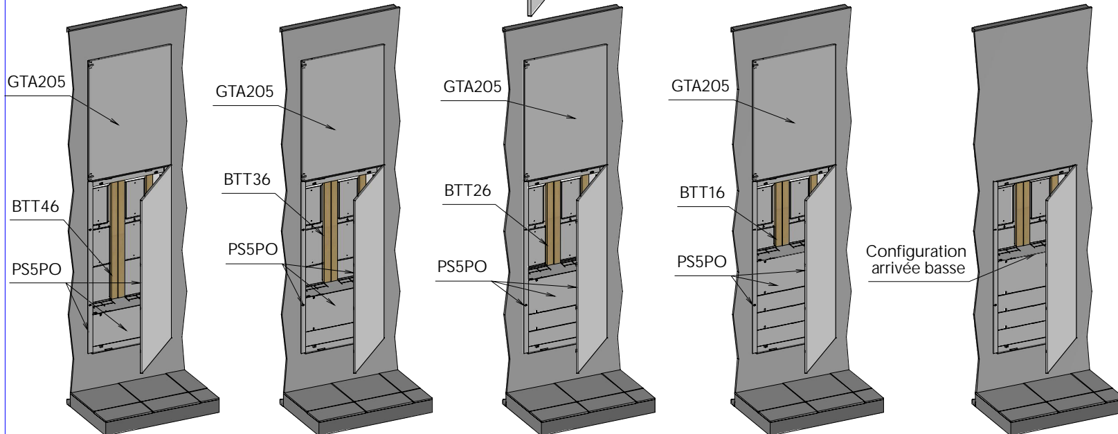
Exemple de mise en oeuvre avec GTA 205
