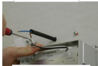
Connexion électrique
