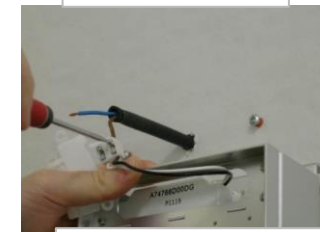
Connexion électrique
