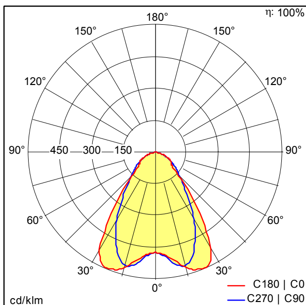
D44421AA_TEC_LED16000-865_L2000_WB_LDE_WH_IP.idt
