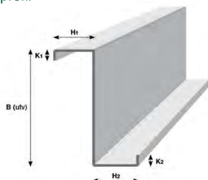
Z-profil
