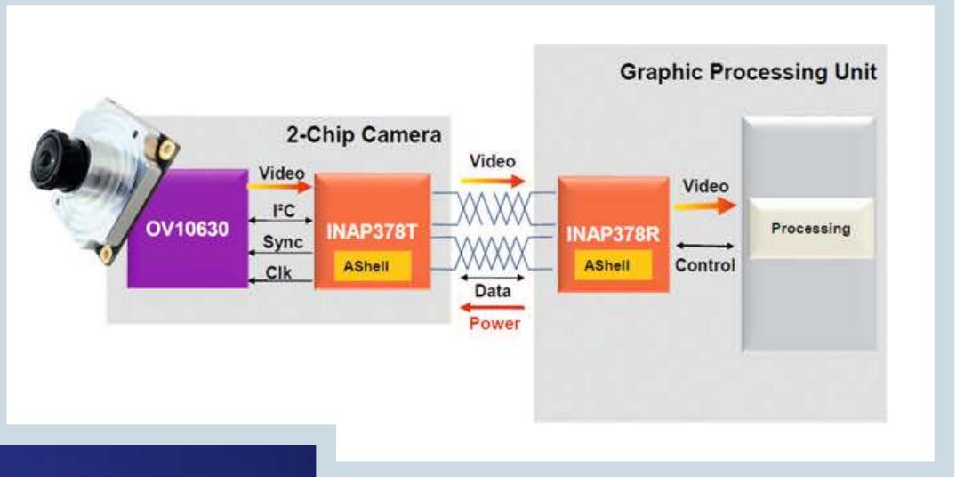
Bild 2: Blockdiagramm des neuen APIX2-Kameralinks mit INAP378T und INAP378R.
