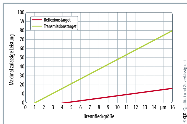
Bild 1. Maximal zulässige Leistung in Abhängigkeit von der angestrebten Auflösung (Brennfleckgröße) für Röhren mit Transmissionstarget (grün) bzw. Reflexionstarget (rot) für den in der Koordinatenmesstechnik wichtigen Bereich (© Werth)
