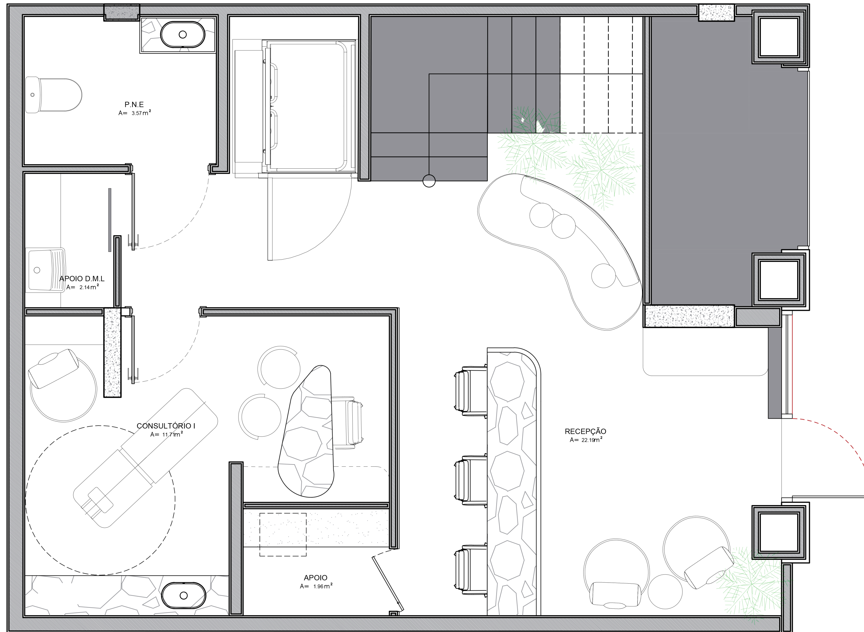
1 PLANTA LAYOUT - TÉRREO ESCALA: 1/25
