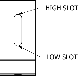
SNAPNRACK 92° L-FOOT
