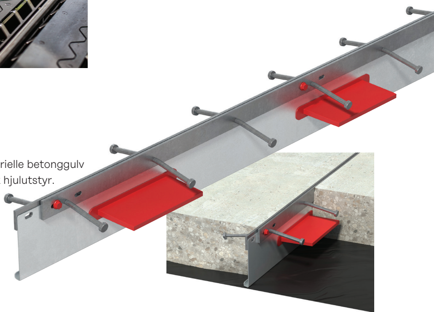
ArmourJoint-Lite® Adjustable
