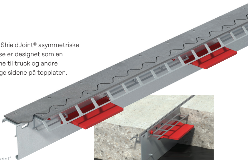
ShieldJoint® Fixed
