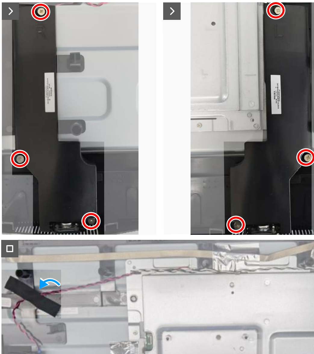
Joonis 10. Kruvide asukohad
