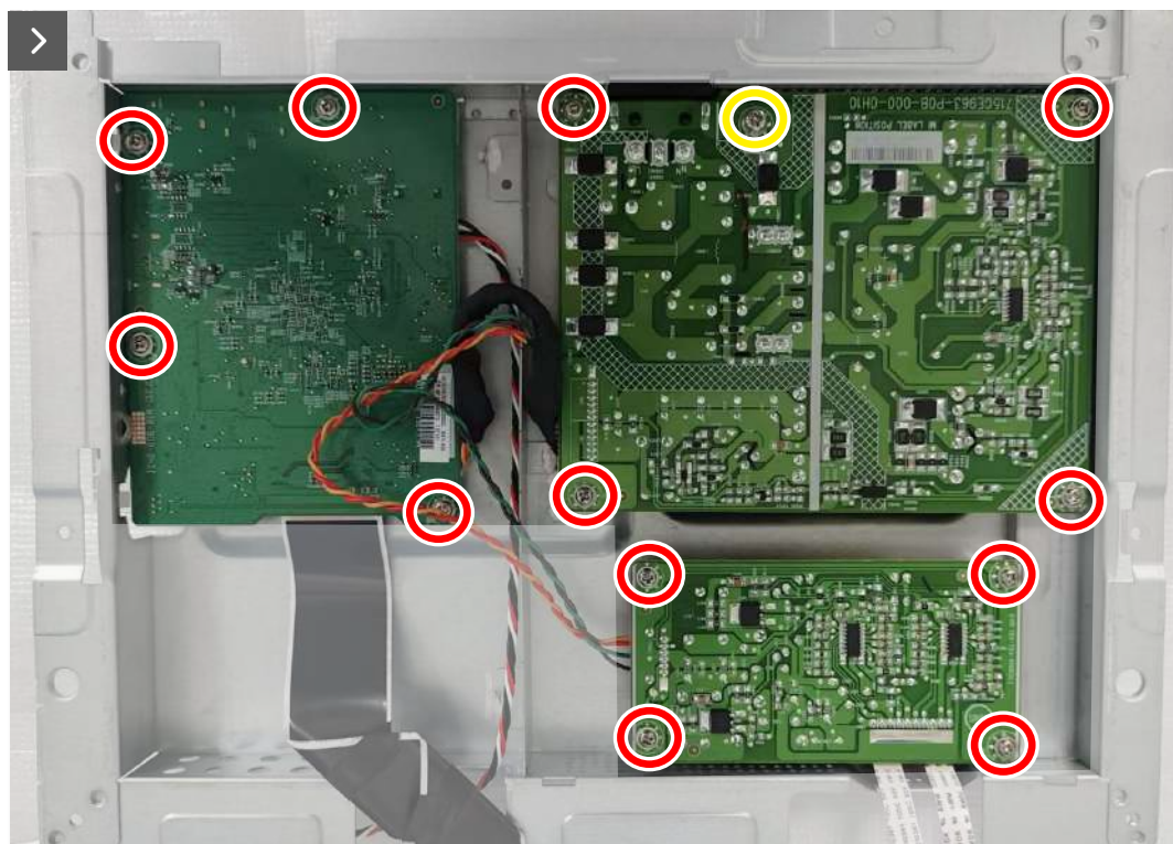
Joonis 22. Kruvide asukohad
