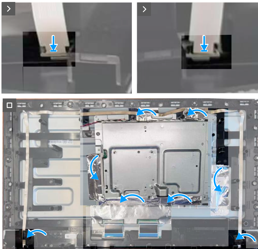
Joonis 16. Valgusriba kaablite ühendamine
