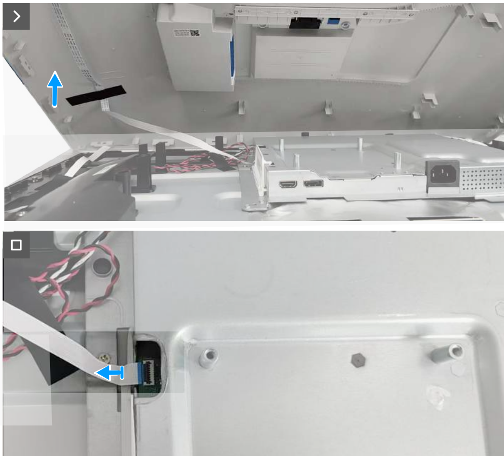
Joonis 4. Klaviatuuriplaadi kaabli lahti ühendamine
