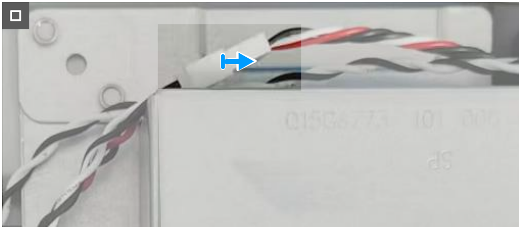
Joonis 8. Kõlari kaabli lahti ühendamine
