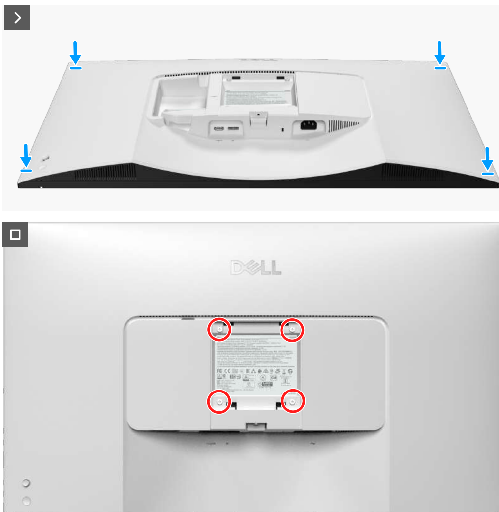
Joonis 6. Kruvide asukohad
