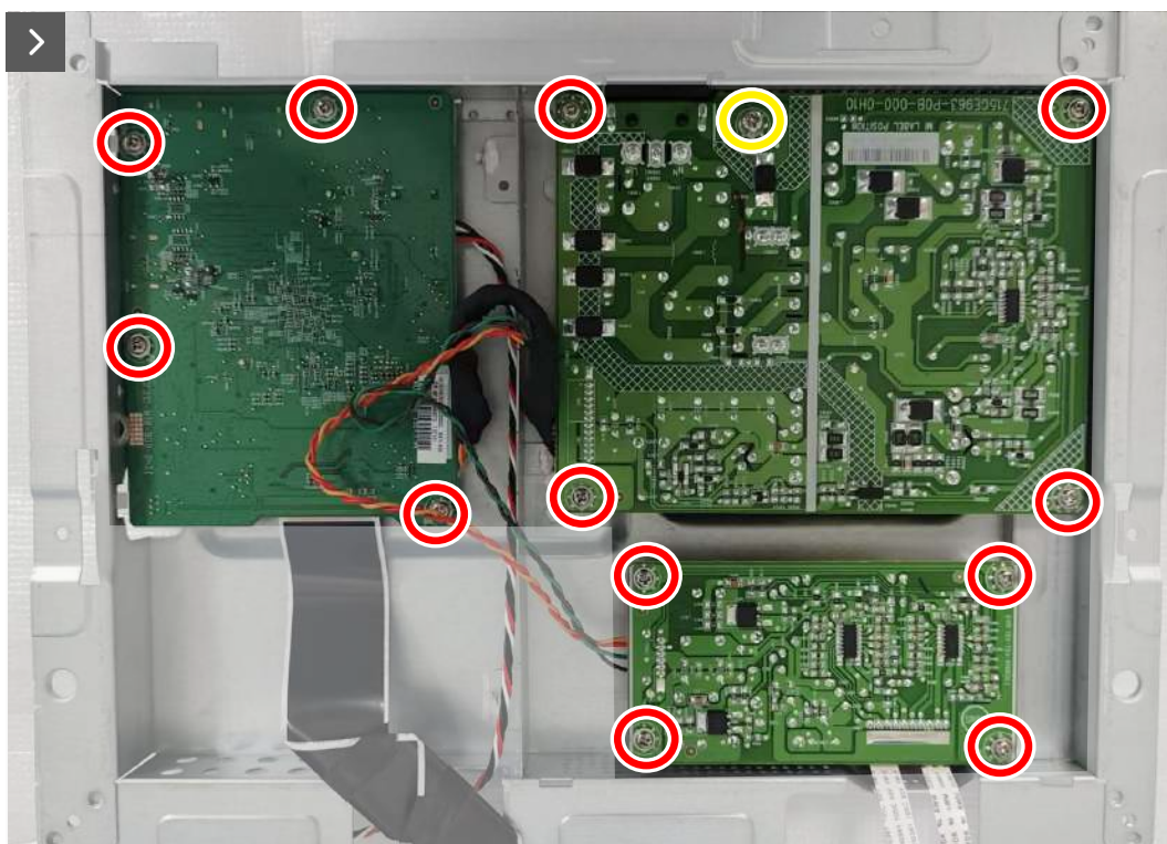
Joonis 19. Eemaldatavad kruvid
