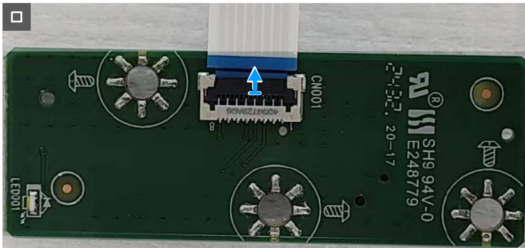
Joonis 28. Klaviatuuriplaadi kaabli lahti ühendamine
