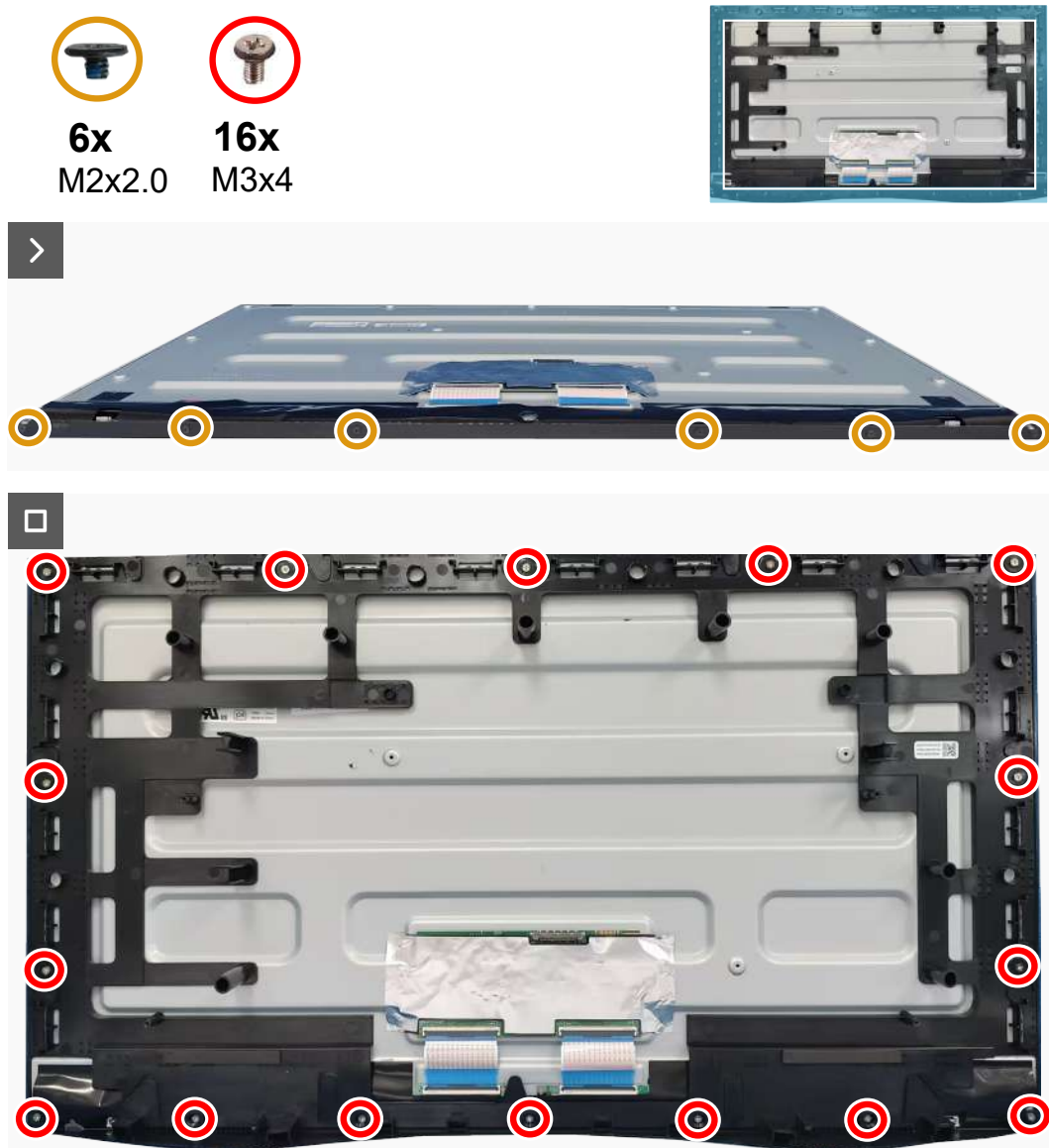
Joonis 26. Kruvide asukohad
