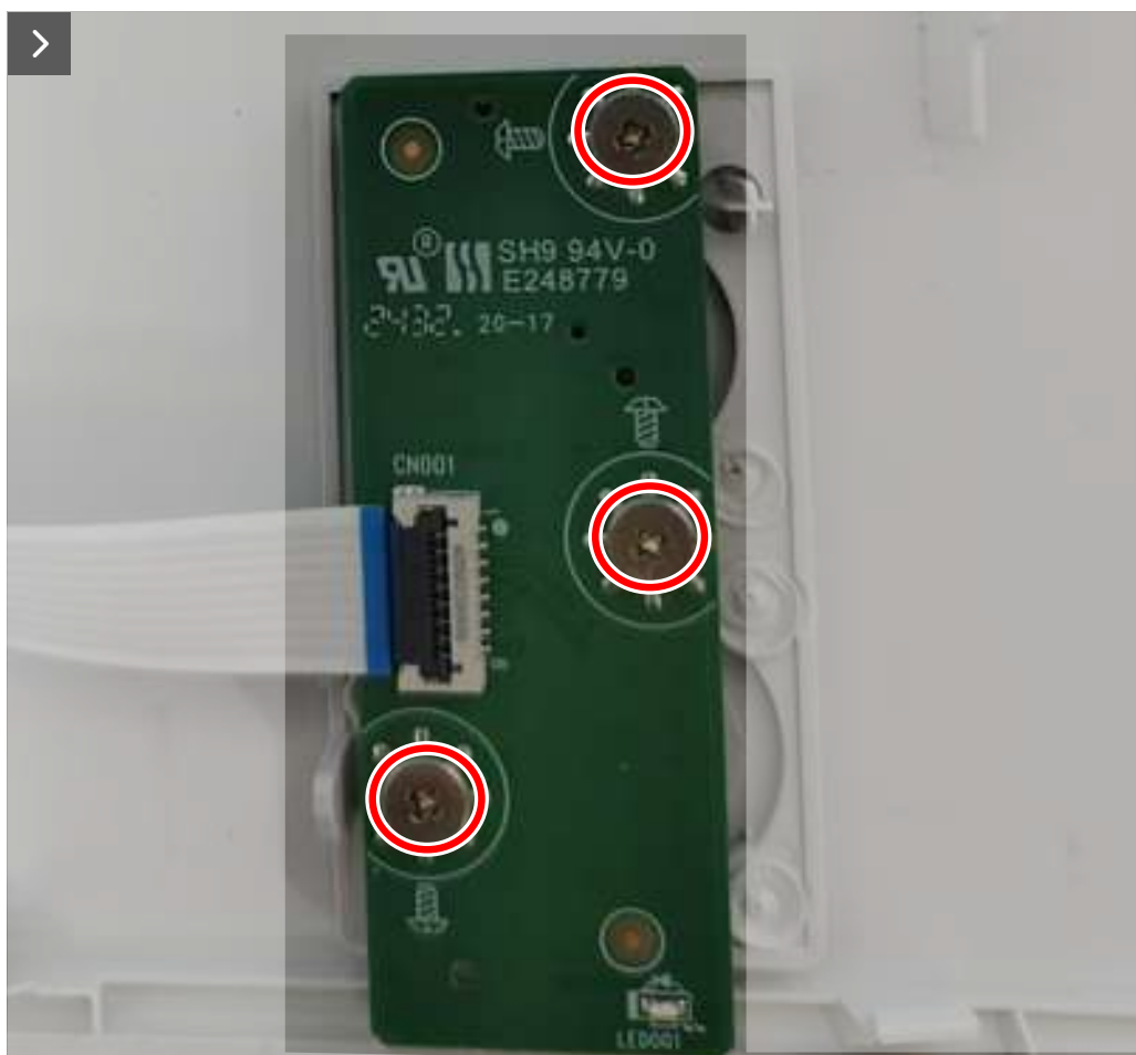
Joonis 27. Eemaldatavad kruvid
