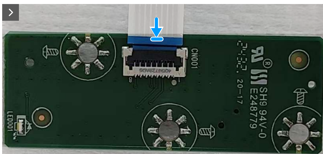
Joonis 29. Klaviatuuriplaadi kaabli ühendamine
