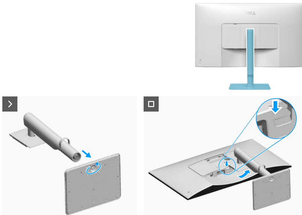
Joonis 2. Jalandi paigaldamine
