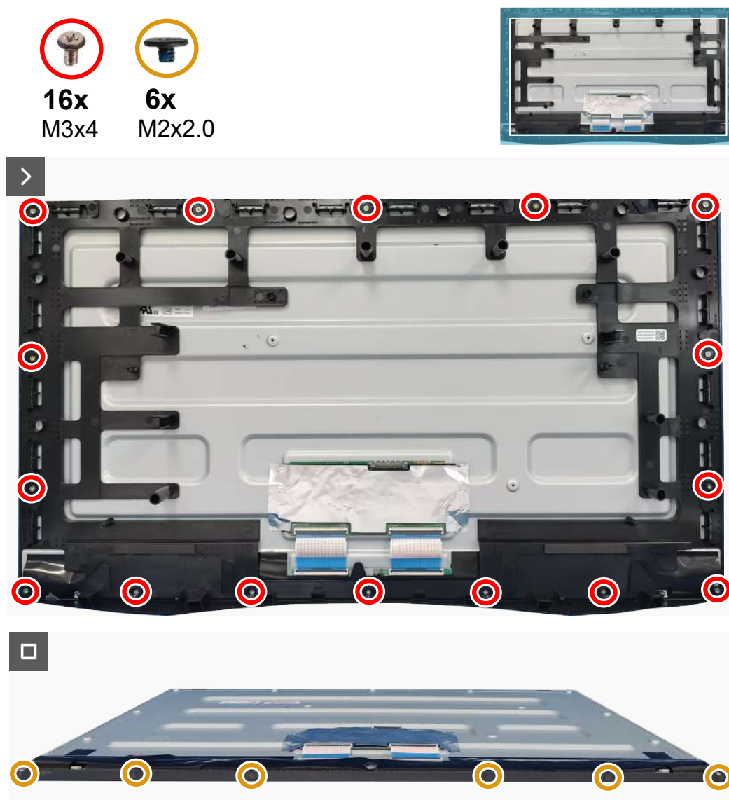
Joonis 25. Eemaldatavad kruvid
