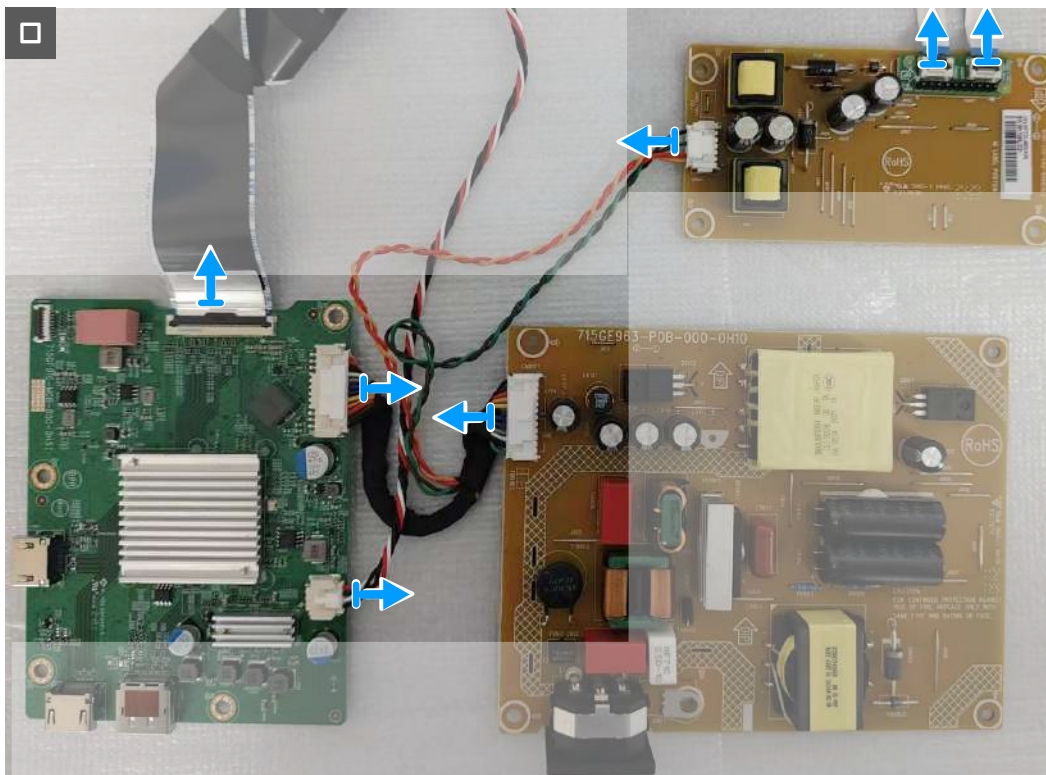
Joonis 20. Kaablite lahti ühendamine
