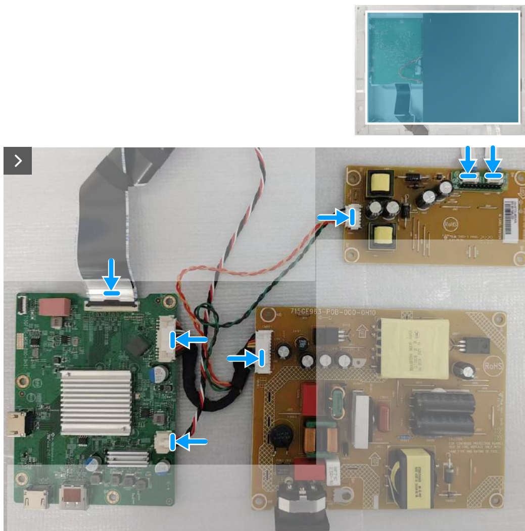
Joonis 21. Kaablite ühendamine
