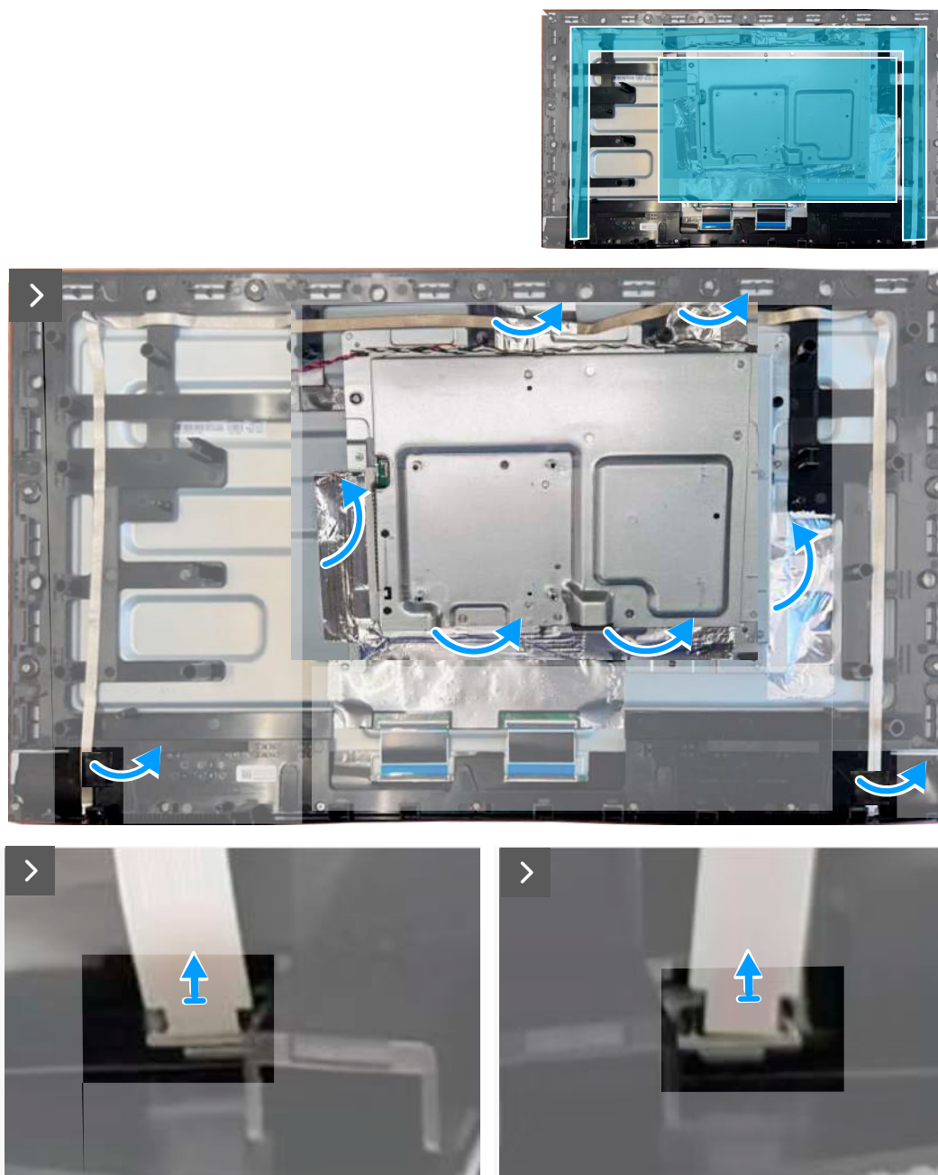
Joonis 11. Valgusriba kaablite lahti ühendamine
