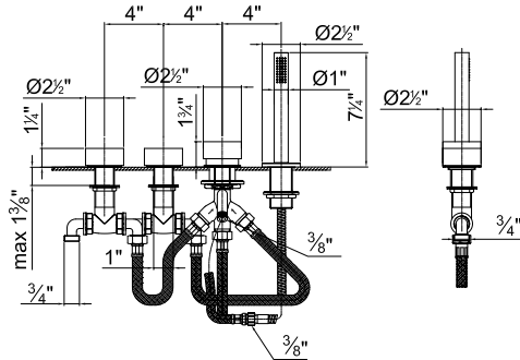
ART. A267U Bath side group / Batería horizontal bañera
