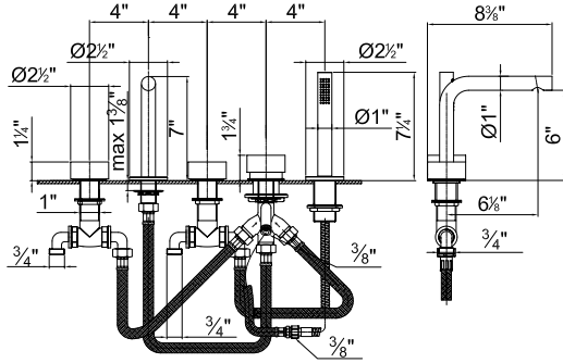
ART. A265U Bath side group with spout / Batería horizontal bañera con cano
