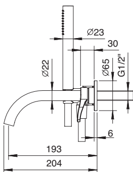
ART. B719B
