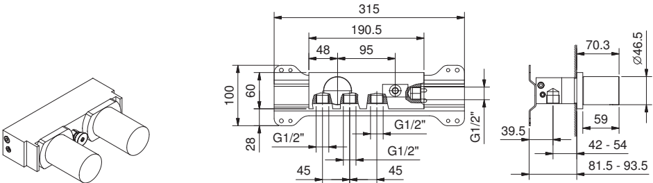
ART. 6185A Parte incasso / Built-in pieces / Partier à encastrer / Eingebaute Stüke / Pedazos incorporados
