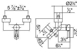
ART. 1815U Bath-tub mixer / Baño ducha
