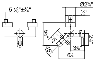
ART. 1818U Bath-tub mixer / Baño ducha
