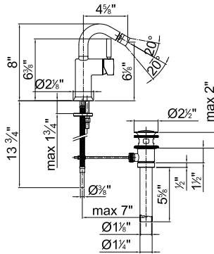
ART. 1808U Bidet mixer / Monomando bidè
