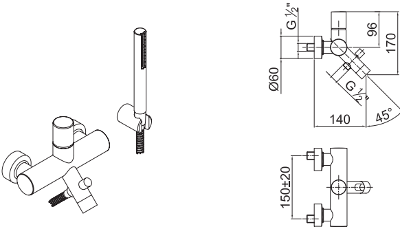
ART. 1615 Vasca esterno / Bath-tub mixer / Bain-douche externe / Aufputz-Wannen / Baño ducha
