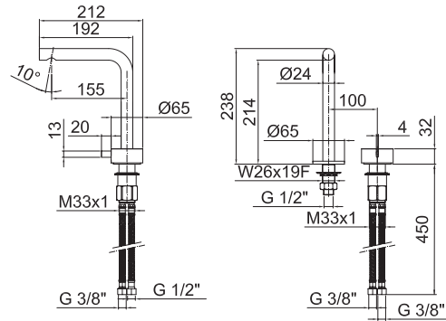
ART. A104WF Gruppo lavabo / Washbasin / Lavabo 1 trous / Waschtischarmatur / Lavabo
